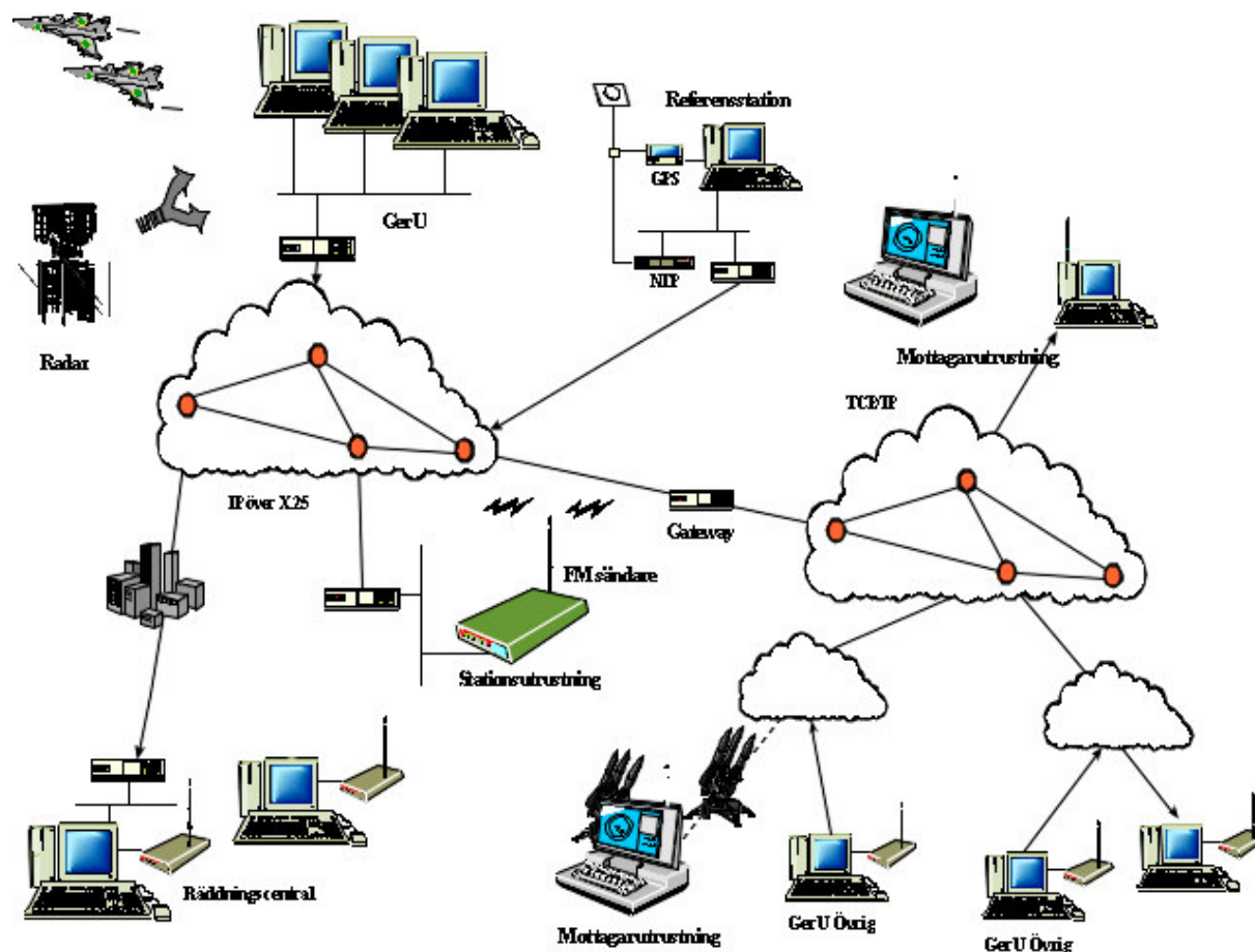
Figur 1 LuLIS Systemskiss
