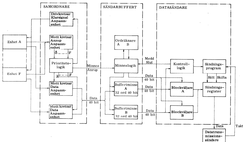
Bild 3. Smalbandsterminal, blockschema
