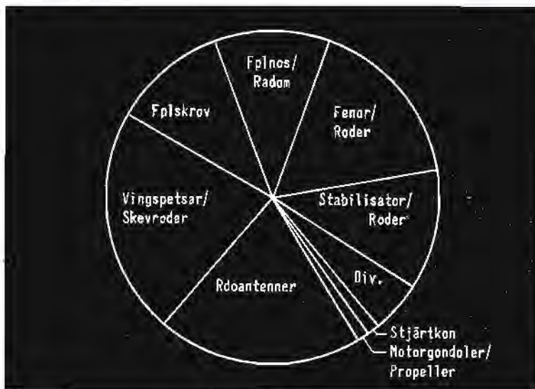
• Fig 6: Beräknad fördelning av träffpunkter vid blixtnedslag i flygplan. Underlaget utgörs av både civila och militära rapporter.
